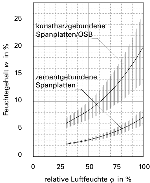
Figur 3 Feuchtegehalt w in % und Streubereich für kunstharzgebundene und zementgebundene Spanplatten und OSB in Abhängigkeit von der relativen Luftfeuchte \phi bei 20 °C
