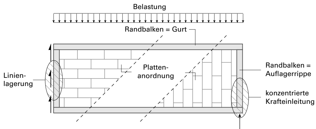
Figur 22 Einleitung der Lasten in die Scheibe und versetzte Plattenanordnung
