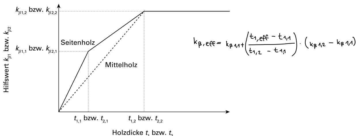
Figur 45 Hilfswert k_{\beta 1} bzw. k_{\beta 2} in Funktion der Holzdicke t_1 bzw. t_2 gemäss den Tabellen 45 und 46 (schematisch)
