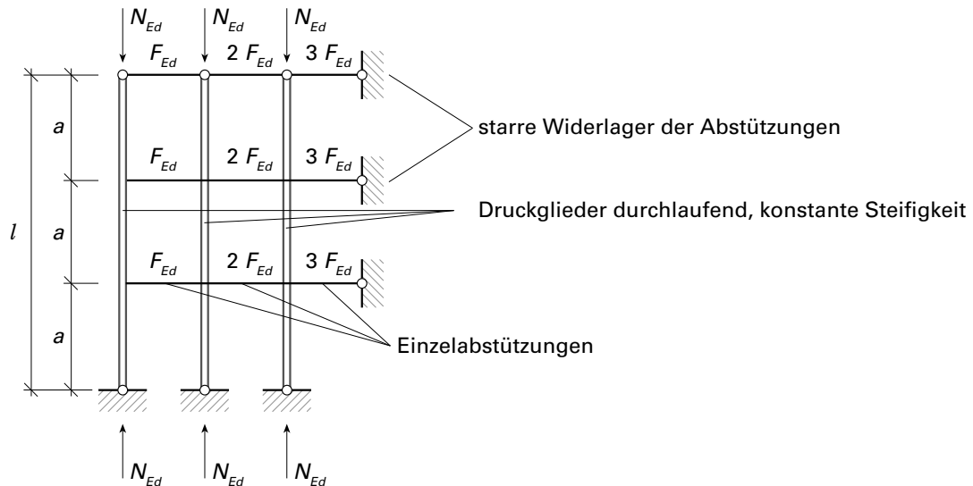
Figur 26 Einzelabstützungen von Druckgliedern bzw. Druckgurten von Biegeträgern
