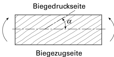
Figur 7 Biegebeanspruchung schräg zur Faserrichtung
