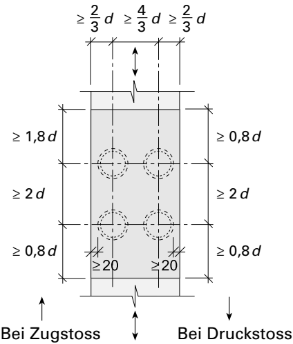
Figur 42 Abstände von Ringdübeln bei Zug- bzw. Druckstoss
