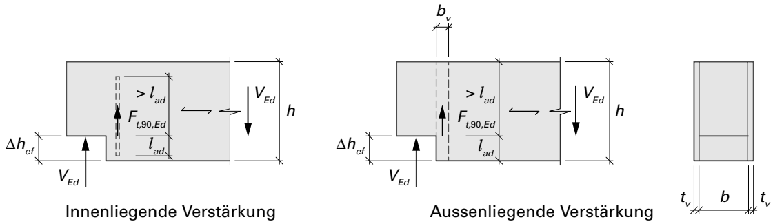
Figur 51 Ausklinkungen mit Verstärkungen
