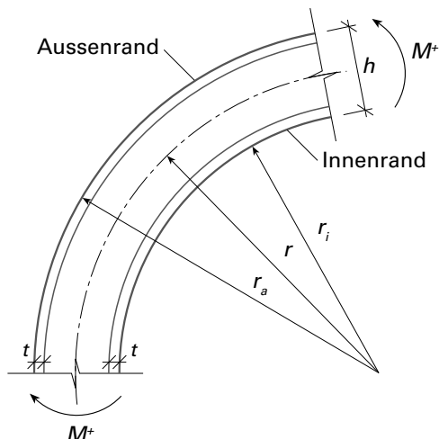
Figur 15 Gekrümmter Träger mit konstantem Querschnitt
