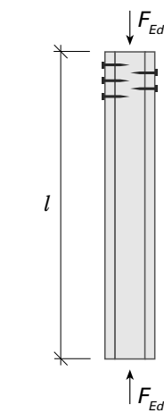
Figur 21a Zusammengesetzte Druckstäbe mit kontinuierlicher, nachgiebiger Verbindung
