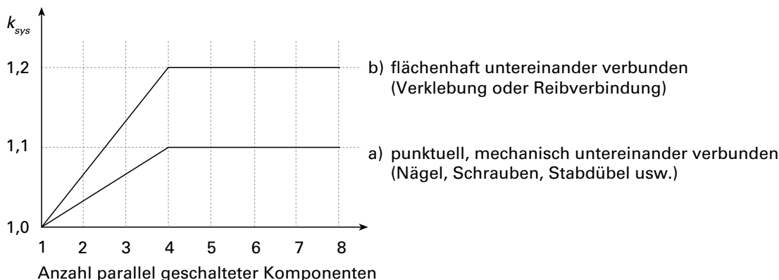
Figur 25 Beiwert zur Erfassung der Systemwirkung k_{sys} für Bauteile aus parallel geschalteten Komponenten
