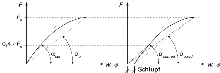
Figur 30 Definition der Verbindungssteifigkeiten \alpha und der verminderten Verbindungssteifigkeiten \alpha_{red} sowie des Schlupfs zur Erfassung der Verformung von Verbindungen
