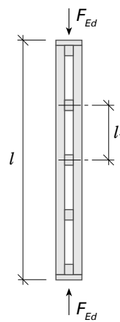
Figur 21b Zusammengesetzte, gespreizte Druckstäbe
