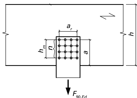
Figur 49 Ansicht mit Bezeichnung der Abmessungen eines Anschlusses mit Querkzugbeanspruchung
