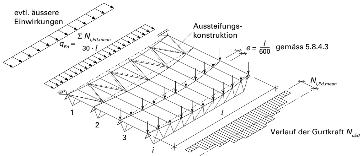
Figur 27 Durch eine Aussteifungskonstruktion seitlich stabilisierte Trägerreihe. Die Gurtkräfte N_{i,Ed} resultieren aus den äusseren, in der Ebene des Trägers i wirksamen Lasten
