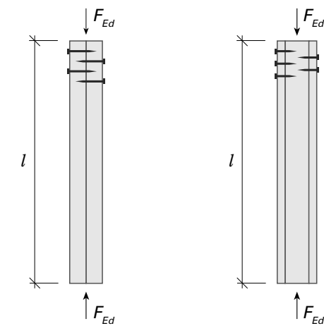
Figur 21a Zusammengesetzte Druckstäbe mit kontinuierlicher, nachgiebiger Verbindung
