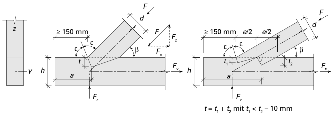
Figur 44 Einfacher und doppelter Versatz
