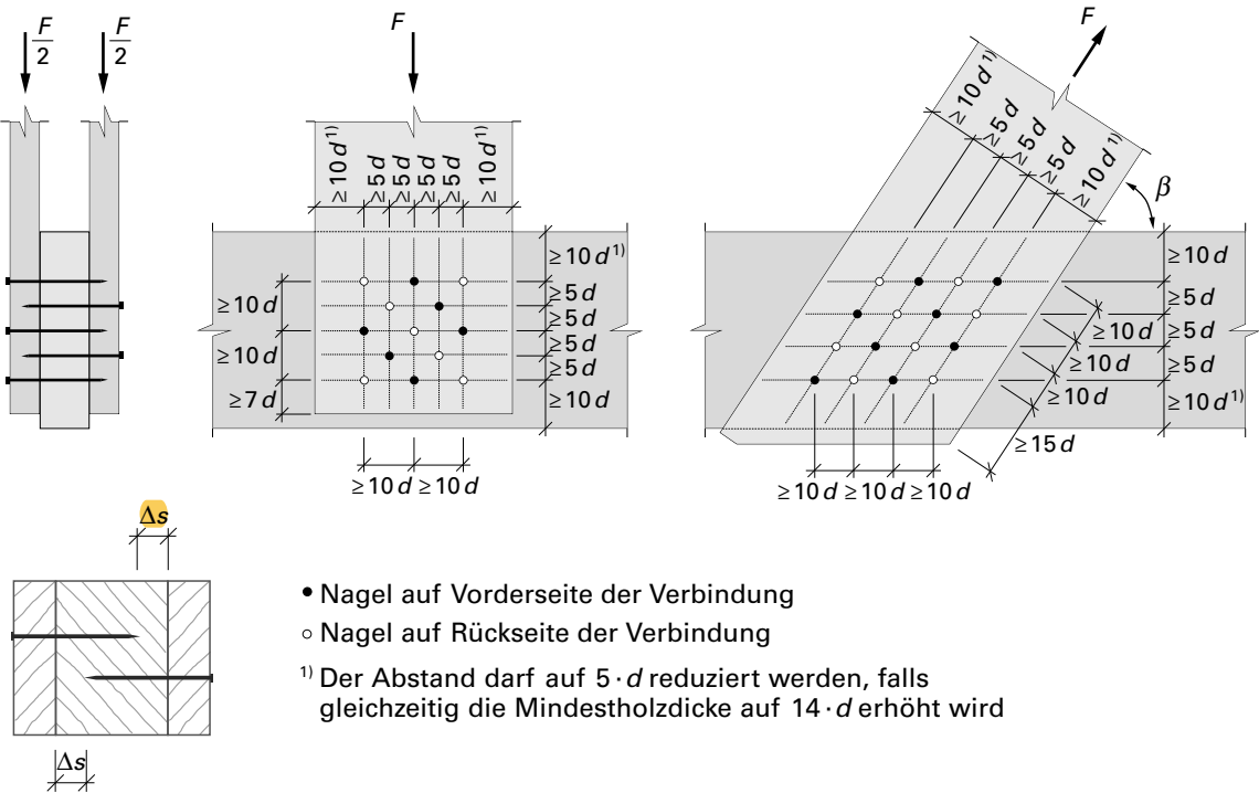
Figur 31 Mindestabstände bei Nageldurchmessern \leq 4 \text{ mm} (für zweischnittige Verbindungen und einschnittige Verbindungen mit \Delta s \leq 5 \cdot d )
