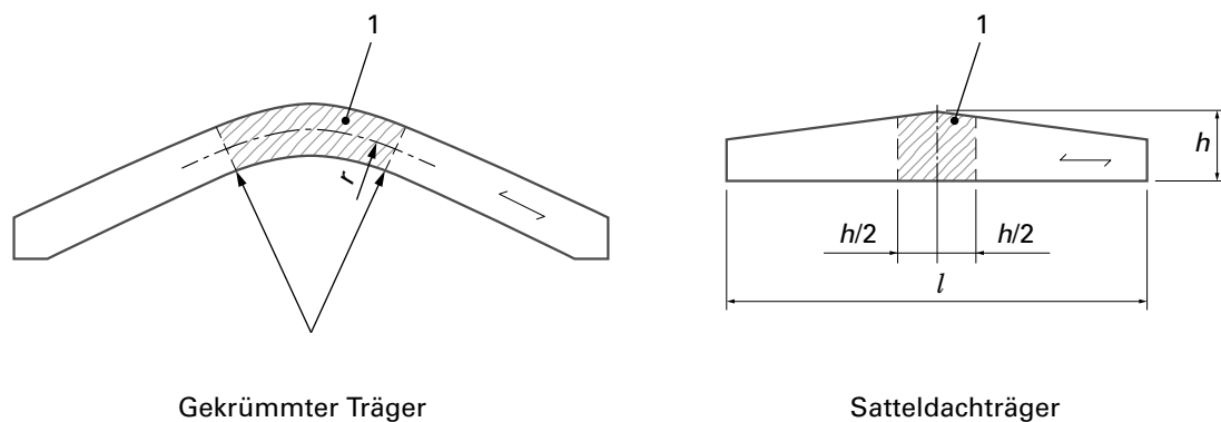
Figur 53 Querzugbeanspruchte Bereiche (1) von gekrümmten Trägern und Satteldachträgern
