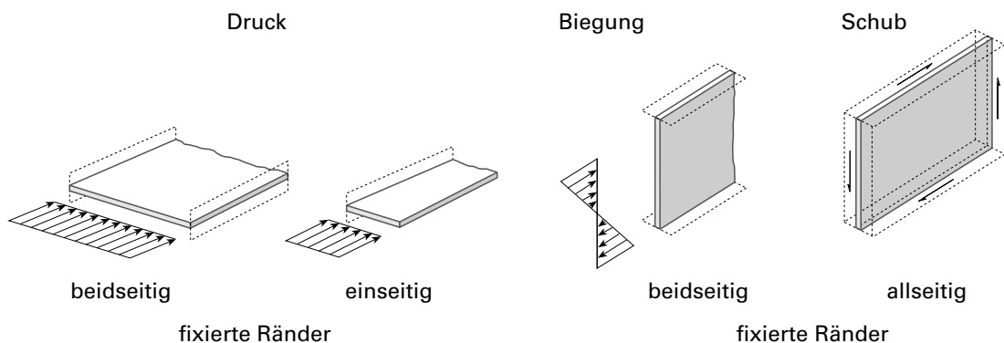
Figur 18 Verschiedene Beanspruchungsarten scheibenförmiger Querschnitte
