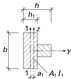
zweiteiliger Querschnitt
