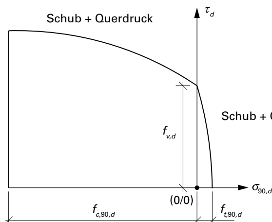
Figur 8 Gleichzeitig wirkende Schubspannungen und Normalspannungen rechtwinklig dazu
