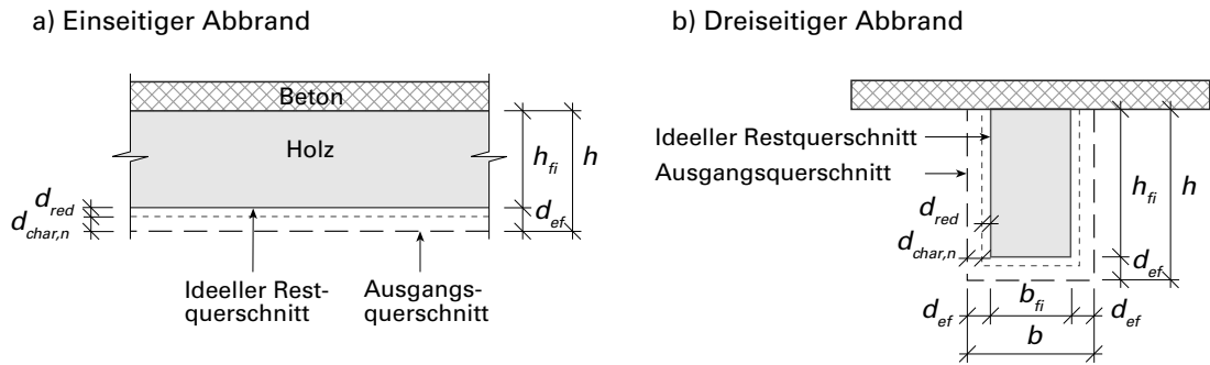
Figur 14 Holz-Beton-Verbunddecken (Querschnitte)
