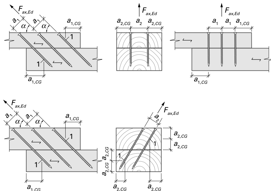
Figur 37 Minimale Abstände für in Schafrichtung beanspruchte Schrauben (1: Schwerpunkt des Gewindeteils im betrachteten Holz)
