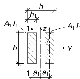
zweiteiliger Querschnitt (m = 2)
