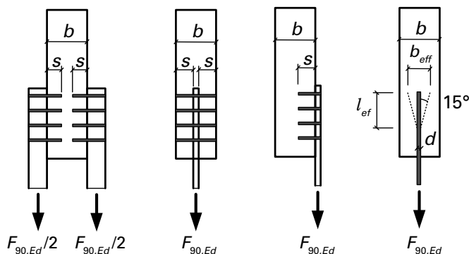
Figur 48 Schnitte mit Bezeichnung der Abmessungen bei beidseitigen, mittigen und einseitigen Anschlüssen mit Querkzugbeanspruchung
