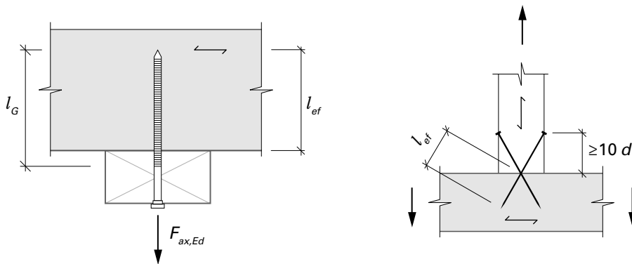
Figur 32 Definition der wirksamen Haft- bzw. Gewindelänge l_{ef} für verschiedene Fälle der Nagelbeanspruchung in Schafrichtung
