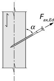
Figur 39 Winkel \alpha zwischen Kraft- und Faserrichtung
