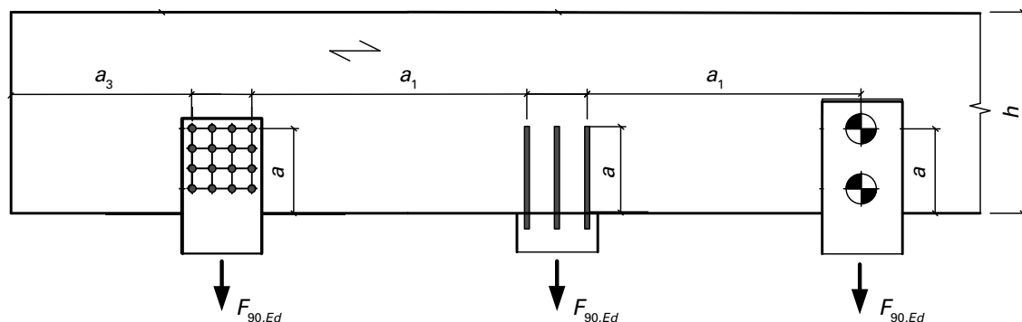
Figur 47 Ansicht mit Bezeichnungen der Lage und der Abmessungen von Anschlüssen mit Querkzugbeanspruchung
