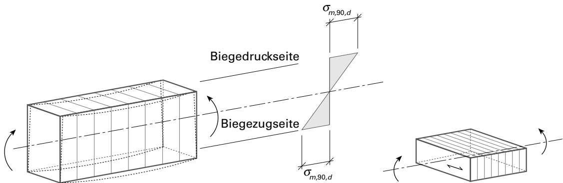
Figur 5 Biegebeanspruchung rechtwinklig zur Faserrichtung
