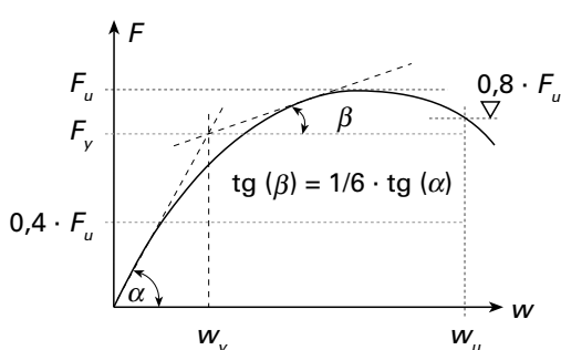
Figur 29 Definition von Steifigkeit und Duktilität
