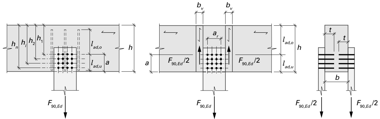
Figur 50 Anschluss mit Querkzugbeanspruchung mit Verstärkungen
