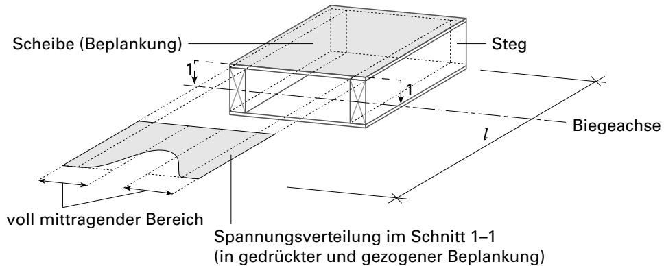
Figur 17 Mittragende Breiten der Beplankung infolge Schubverformung bei Biegung mit Querkraft
