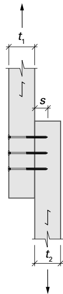
Figur 35 Einschnittige Holz-Holz-Verbindung
