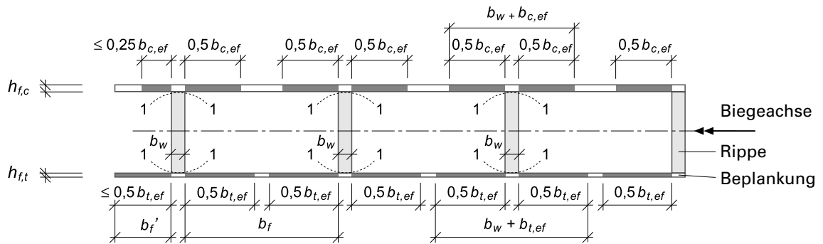
Figur 19 Beidseitig beplanktes Tafелеlement
