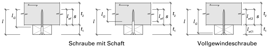
Figur 38 Wirksame Gewindelänge l_{ef} auf der Seite der Schraubenspitze
