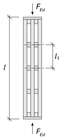
Figur 21b Zusammengesetzte, gespreizte Druckstäbe
