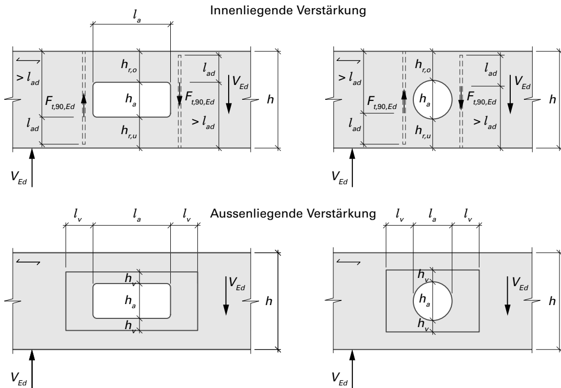
Figur 52 Durchbrüche mit Verstärkungen
