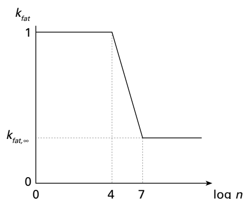
Figur 12 Reduktionsbeiwert im Ermüdungsnachweis k_{fat}
