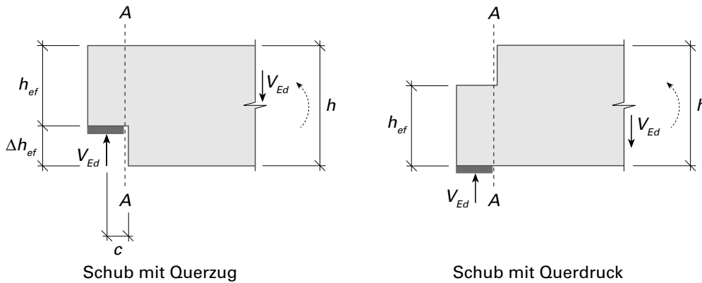
Figur 16 Beanspruchungsarten von Ausklinkungen
