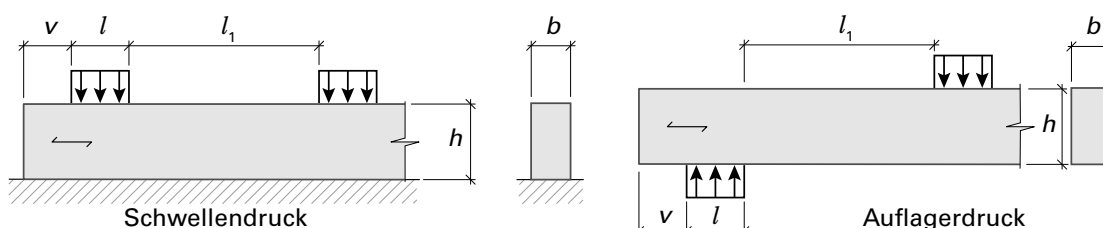
Figur 46 Druck rechtwinklig zur Faserrichtung des Holzes
