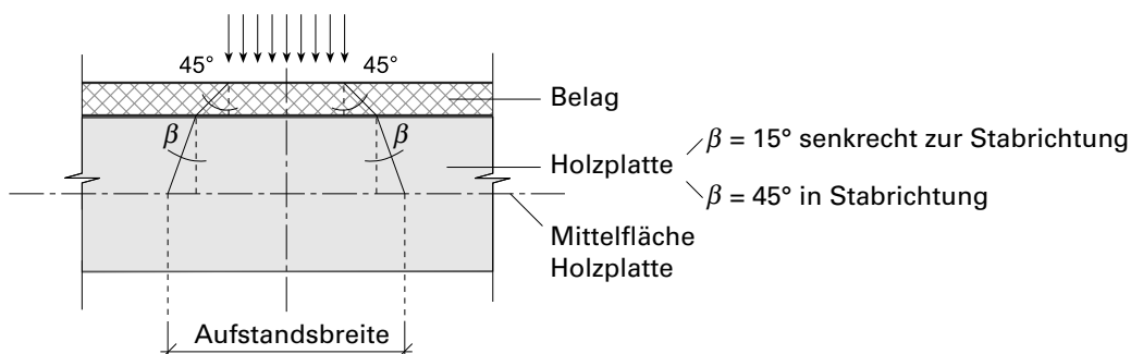
Figur 24 Bestimmung der Aufstandsbreite
