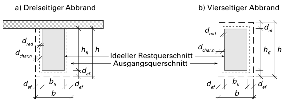
Figur 13 Bestimmung des ideellen Restquerschnitts im Brandfall
