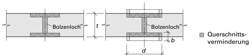
Figur 40 Querschnittsverminderung bei Einpress- und Einlassdübeln
