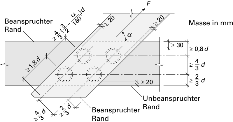
Figur 41 Abstände von Ringdübeln
