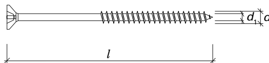
Figur 34 Holzschrauben mit gewalztem oder geschmiedetem Gewinde
