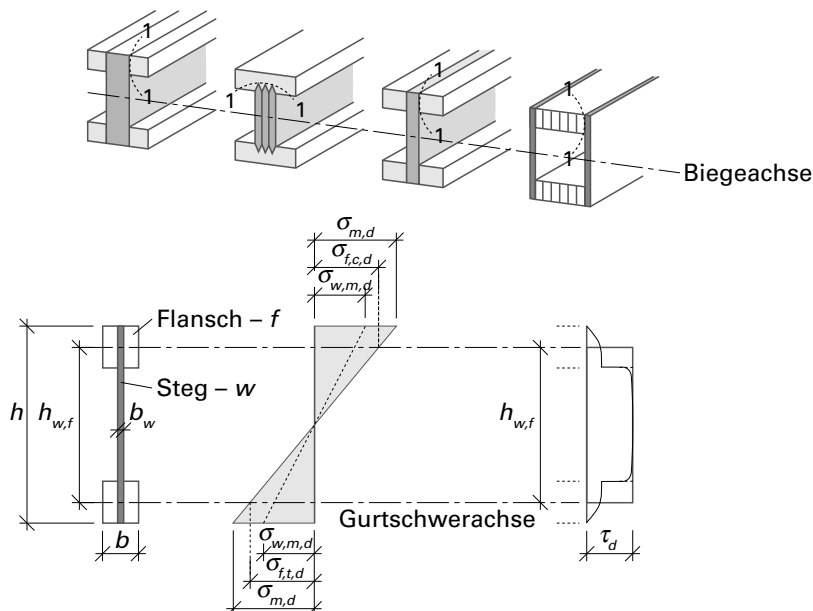
Figur 20 Ausbildungsformen und Spannungsverlauf in Stegträgern infolge Biegung und Querkraft
