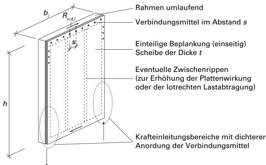
Figur 23 Individuelles Wandscheibenelement
