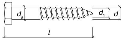
Figur 33 Holzschraube mit geschnittenem Gewinde nach DIN 7998
