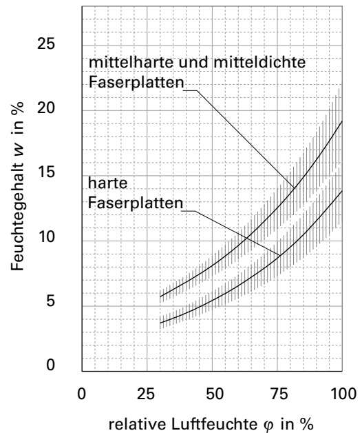
Figur 4 Feuchtegehalt w in % und Streubereich für Faserplatten in Abhängigkeit von der relativen Luftfeuchte \phi bei 20 °C
