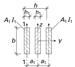
dreiteiliger Querschnitt (m = 3)
