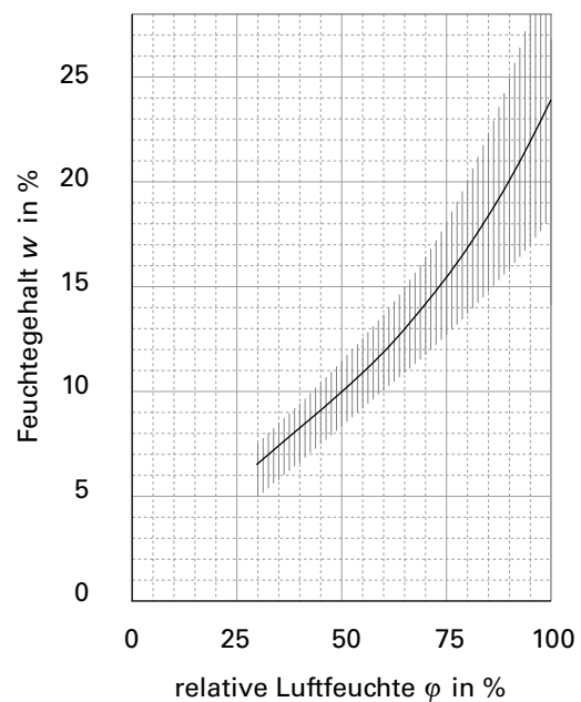
Figur 2 Feuchtegehalt w in % und Streubereich für Brettschichtholz, Balkenschichtholz, ein- und mehrlagige Massivholzplatten, Brettsperrholz, Furnierschichtholz und Furniersperrholz in Abhängigkeit von der relativen Luftfeuchte \phi bei 20 °C
